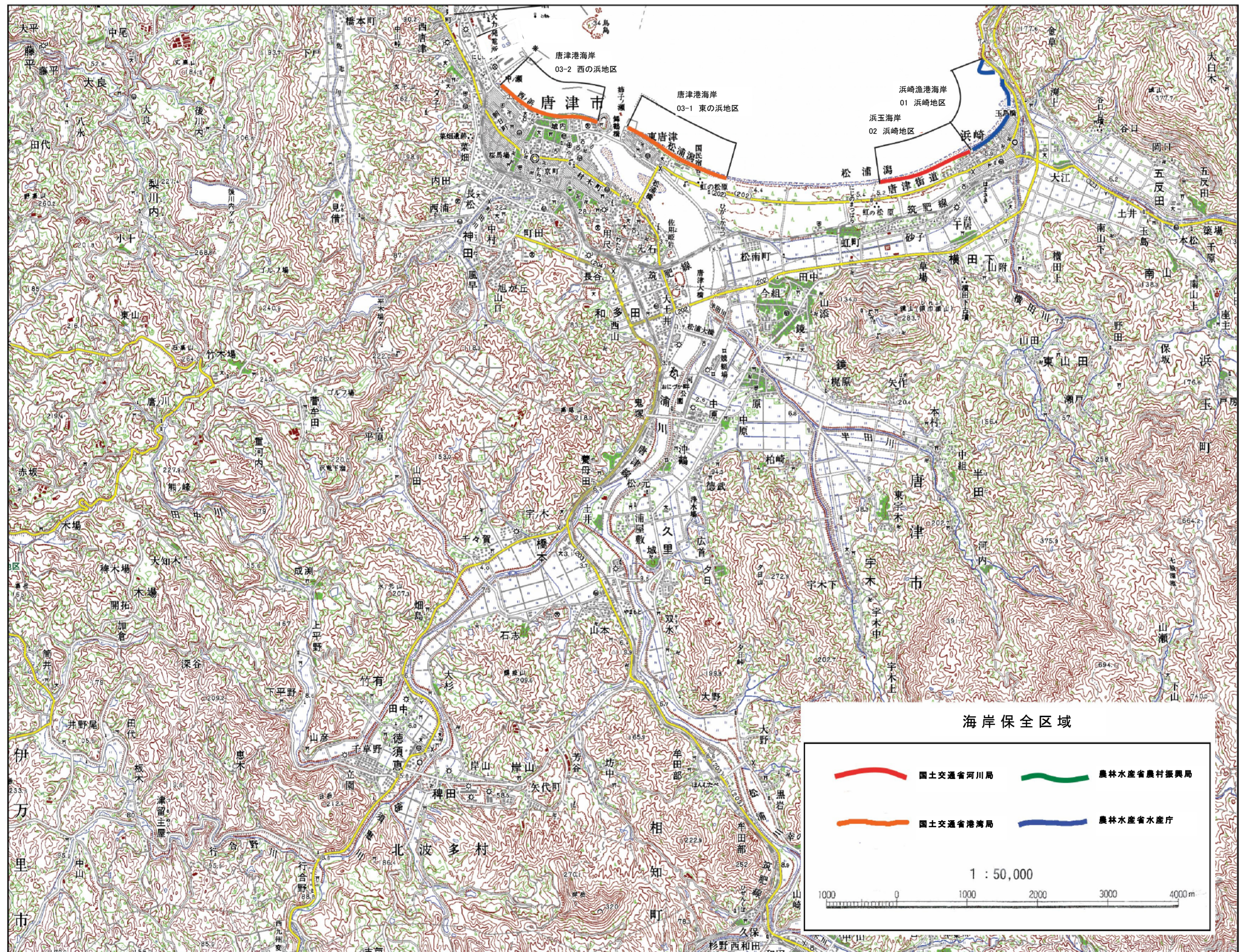
図2.1 海岸保全施設の配置
