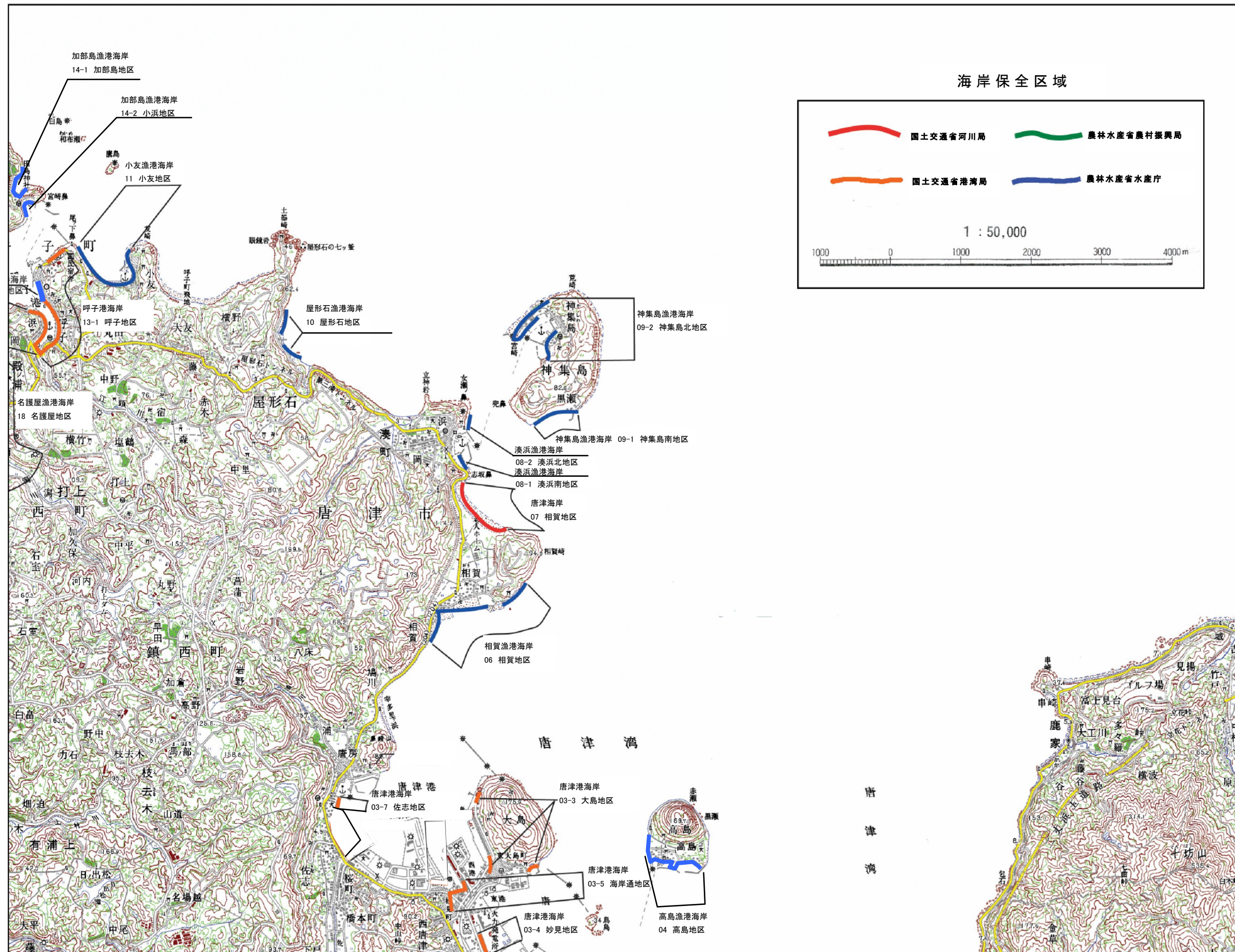
図2.1 海岸保全施設の配置
