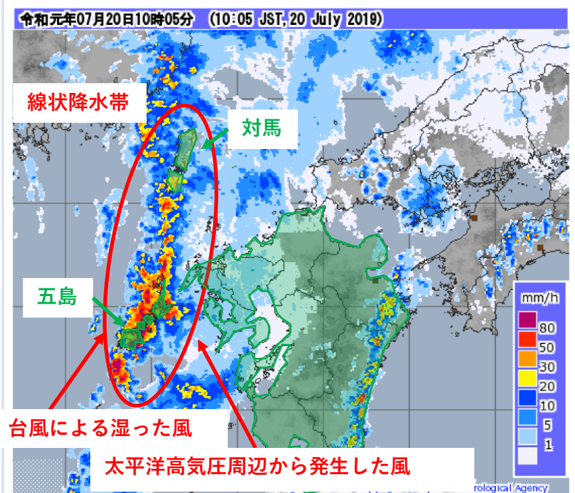
図-1 令和元年7月20日10時05分時点線状降水帯 出典：気象庁ホームページより
