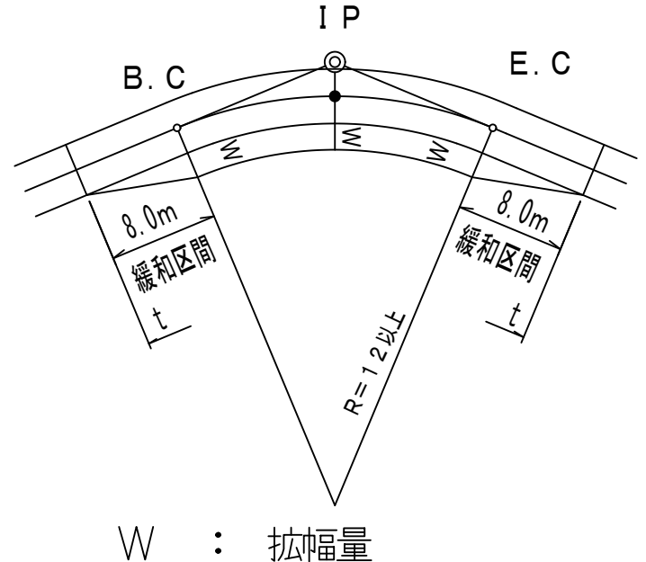
図-2 曲線半径、拡幅、緩和区間
