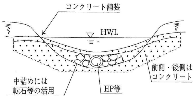
参考図-2 洗越工
