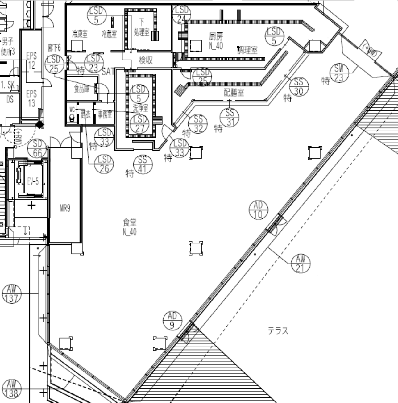
厨房・食堂建具配置図
