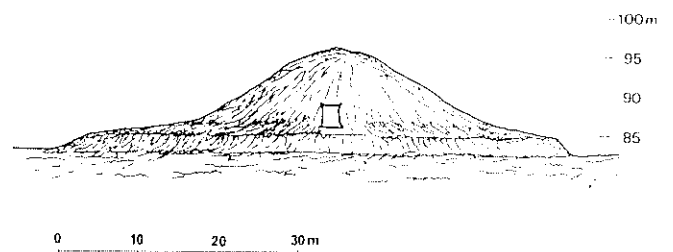
図6 笹塚古墳墳丘復原図
