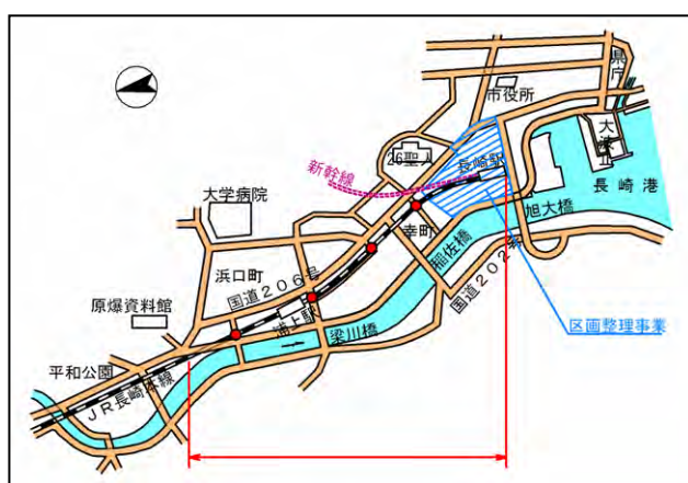
図- 4 <J R長崎本線連続立体交差事業>
