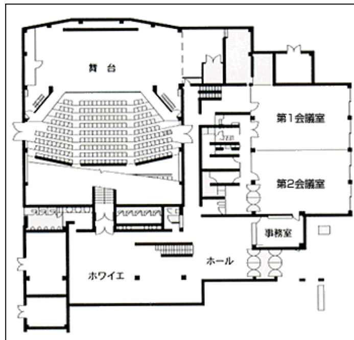
平面図(1階)
