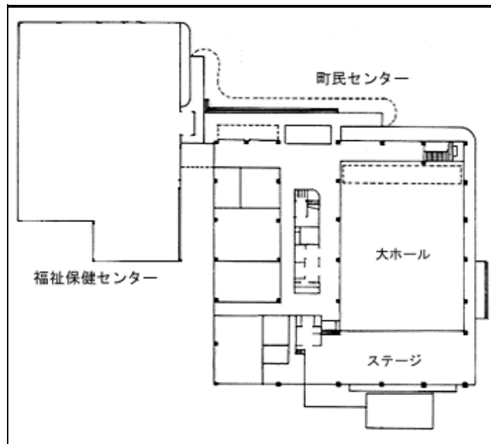
平面図(1F)
