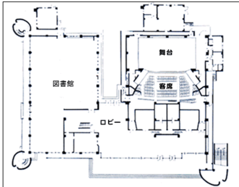
平面図(一階)
