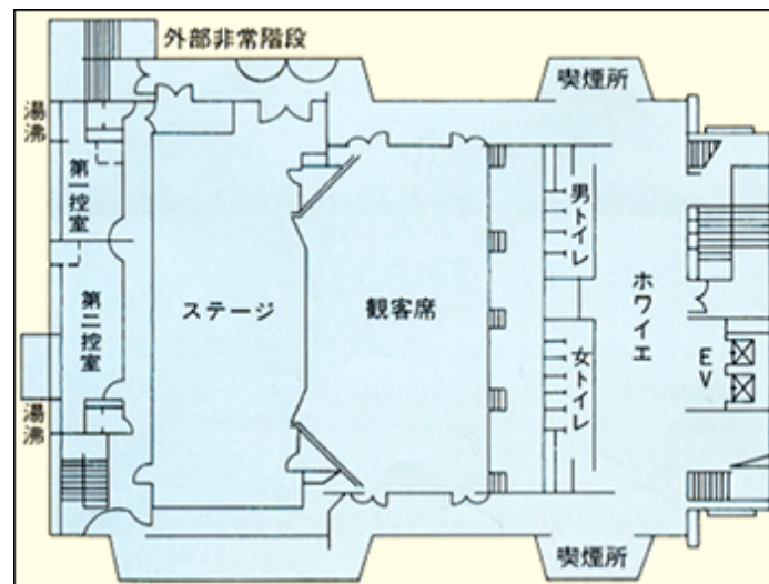
平面図(5階)
