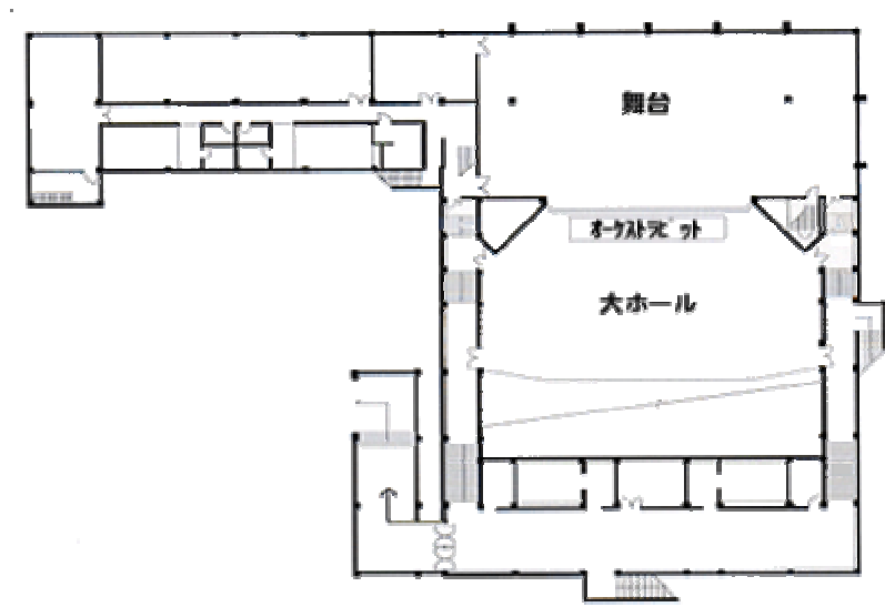
平面図(地階)
