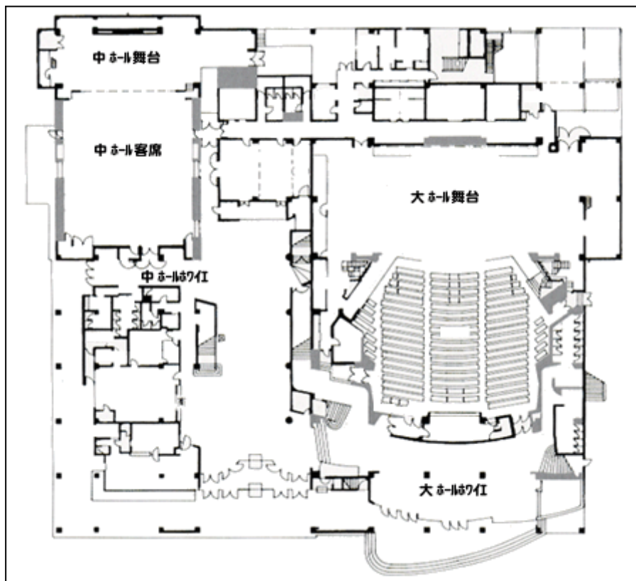
平面図(1階)
