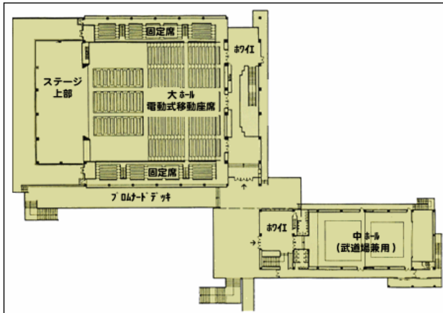
平面図(2階)
