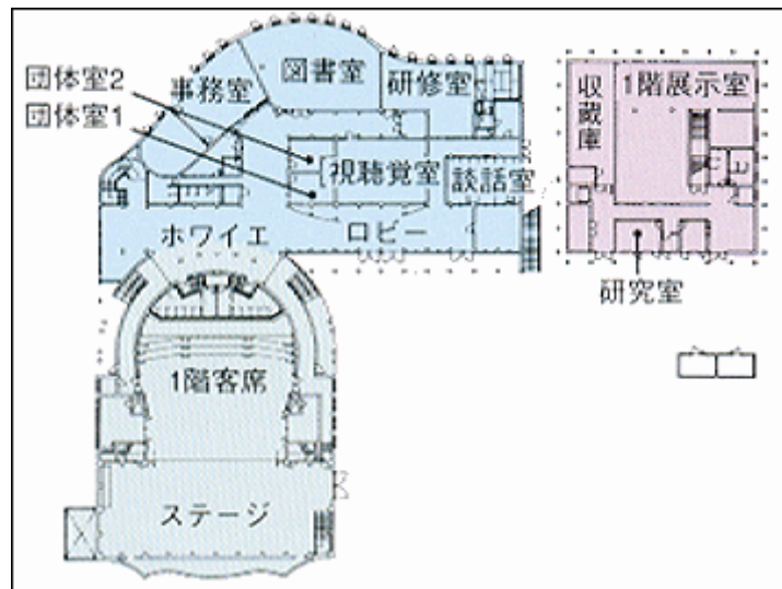
平面図(1階)
