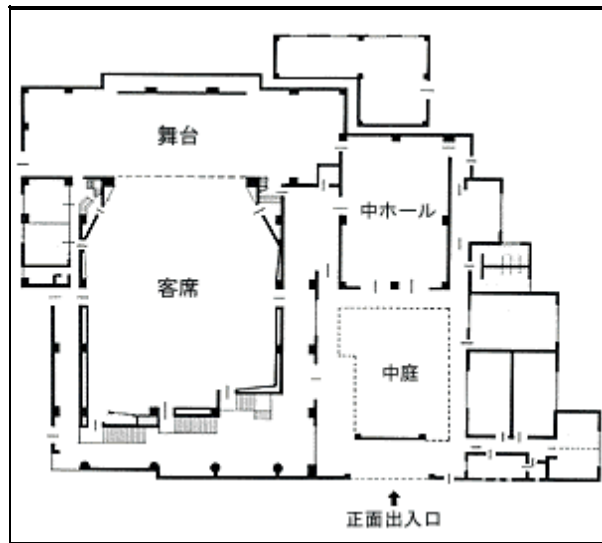
佐々町文化会館 ホール(平面図)
