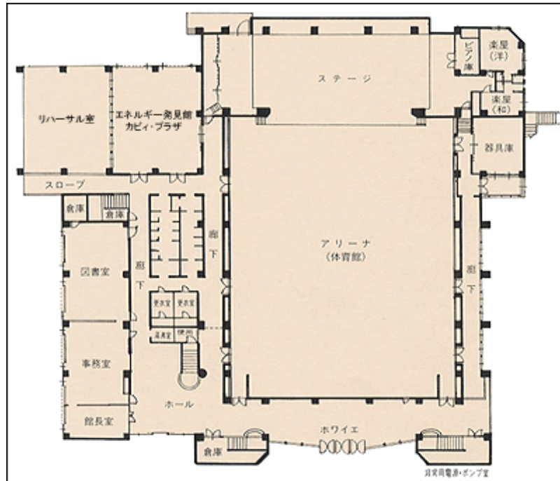
平面図(1階)
