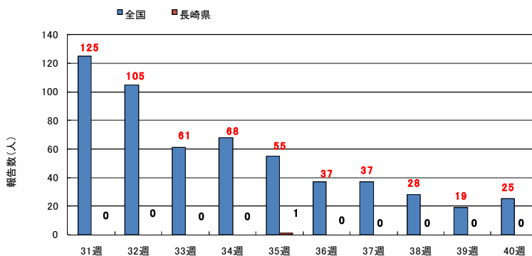
報告週（2013年31週～第40週まで） 全国と長崎県の風疹の報告数の推移
