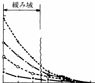
図 15 緩み域の推定 (例)
