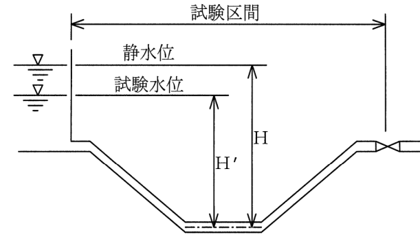
図 - 4 試験水頭のとり方
