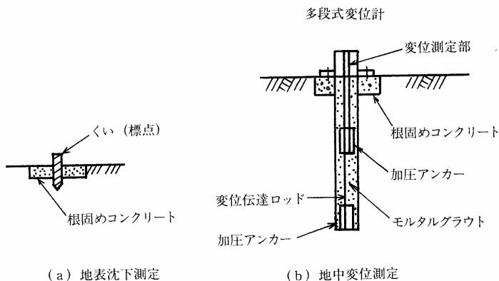
図-20 地表沈下測定構造
