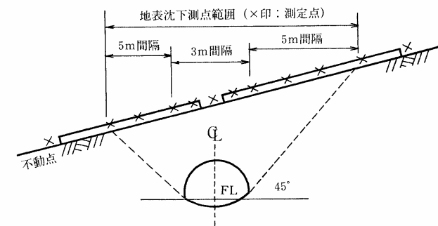
図-22 地表沈下測点の配置
