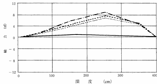
図-18 ロックボルト軸力分布図(例)
