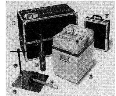
図-4 計器の構成例(透過型)
