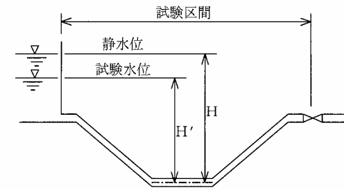
図 - 4 試験水頭のとり方
