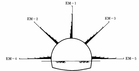
図 12 地中変位計の設置(例)
