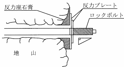
図-28 反力座の設置
