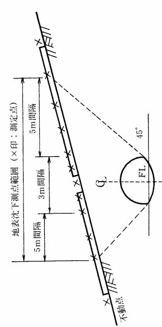
図-22 地表沈下測定の配置
