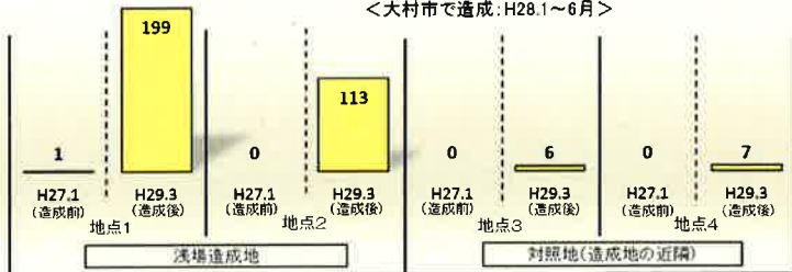
再生砂による浅場造成に伴うアサリ出現個体数(30×30cm範囲内) <大村市で造成: H28.1~6月>
