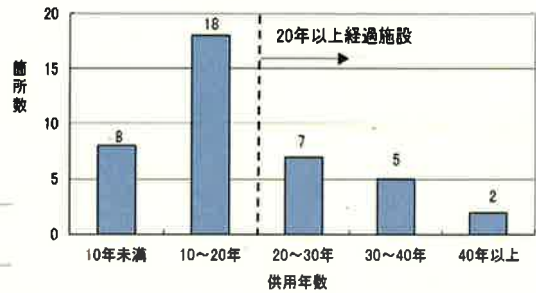
供用年数別の下水処理場
