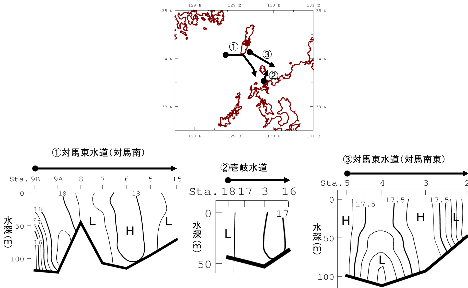
図1 水温鉛直断面図
