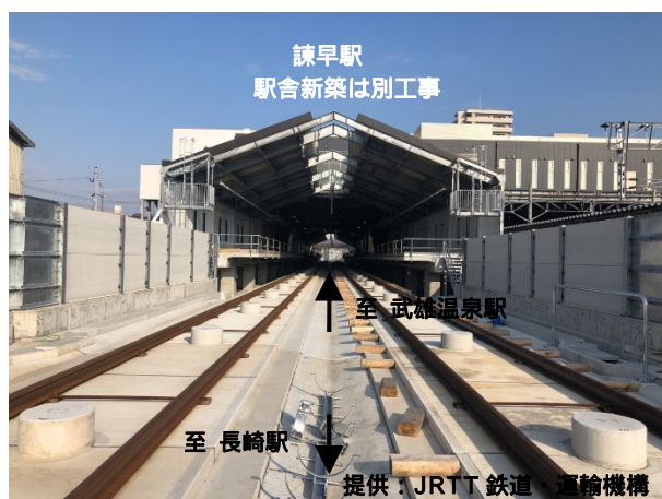
竣工した「諫早駅路盤」工区 （諫早駅部）
