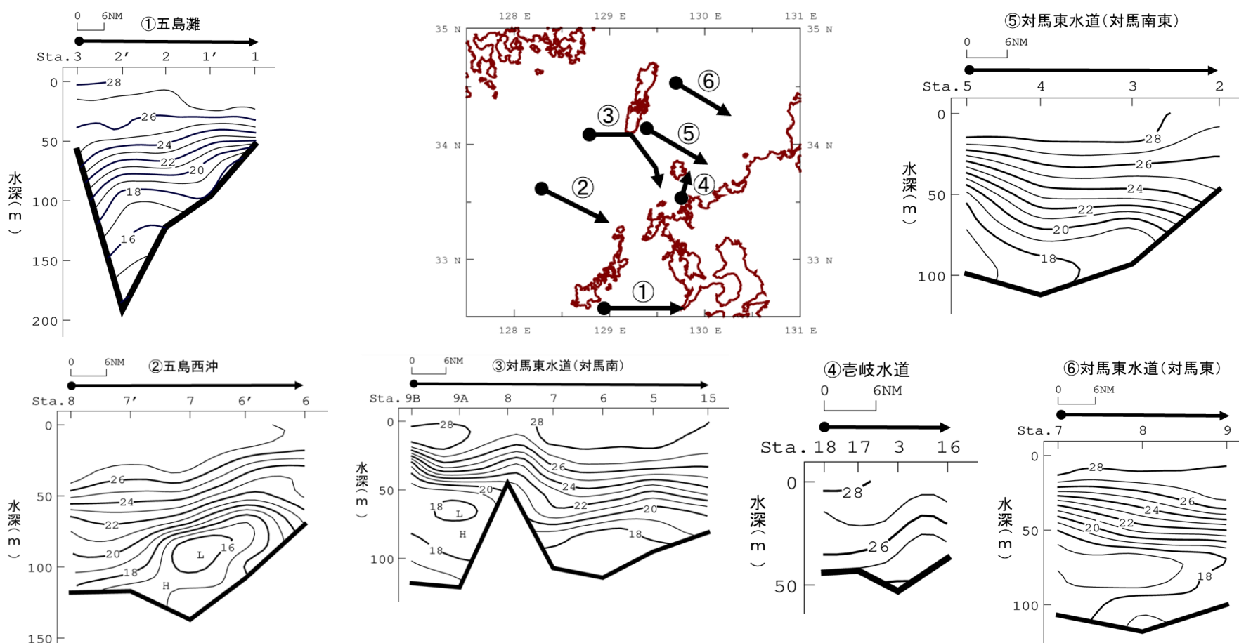
図1 水温鉛直断面図
