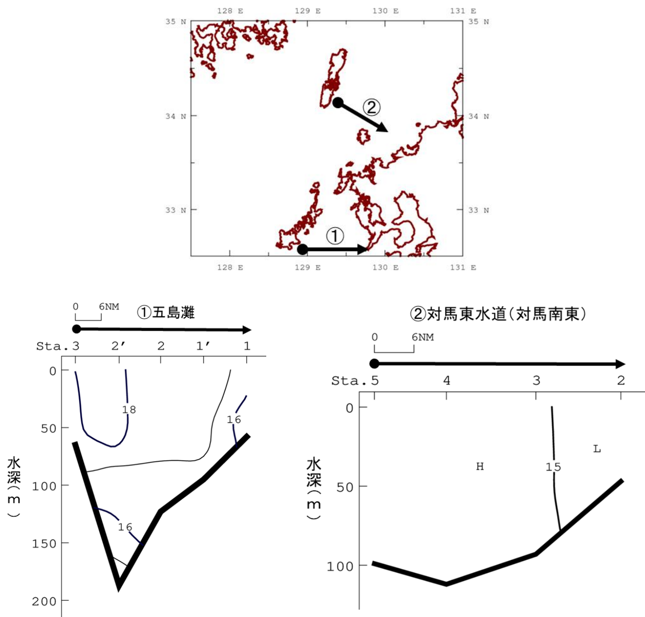
図1 水温鉛直断面図
