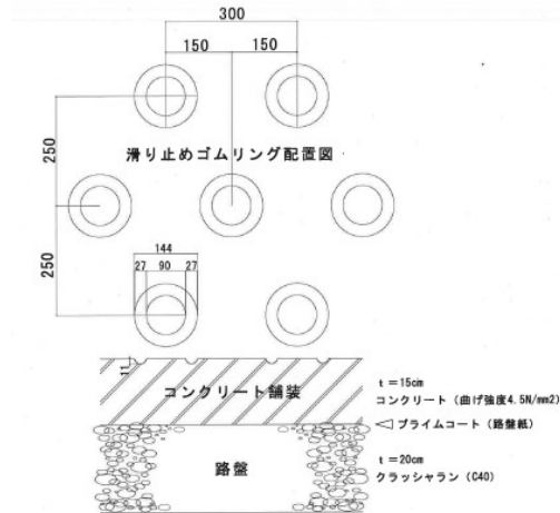
【滑り止め舗装参考図】
