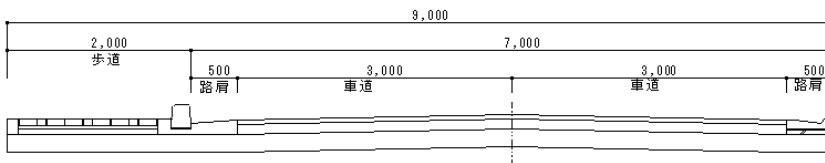
片側歩道（W=2m）を設置する場合：道路幅員9m
