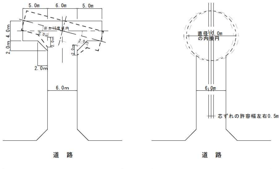
【終端部に設ける転回広場の形状】 ※広幅員道路の場合は別途協議を必要とする。
