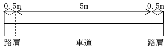
6.0m道路の幅員構成
