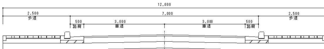
両側歩道（W=2.5m）を設置する場合：道路幅員12m
