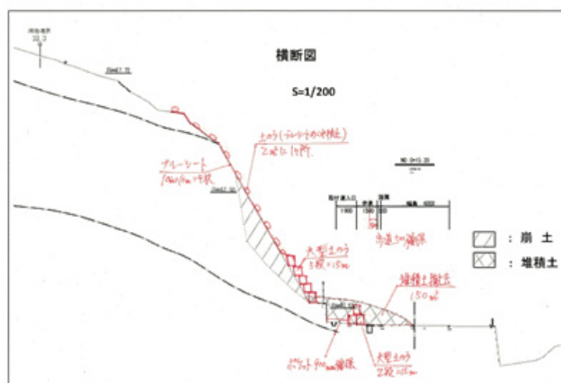
▲Aチーム検討結果（計画横断面図）
