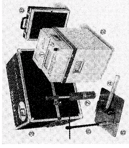
①計器本体 ②標準体 ③収納箱 ④鉄ハンマー ⑤ベースプレート ⑥線源棒 ⑦線源筒 ⑧付属品収納箱
