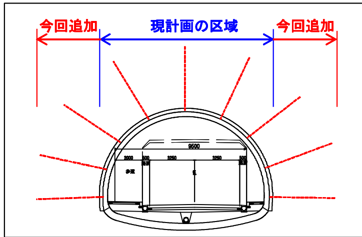
【A - A'断面】 (ロックボルト 4m区間)
