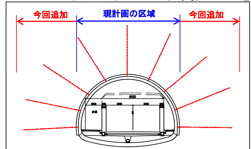
【B - B'断面】 (ロックボルト 6m区間)
