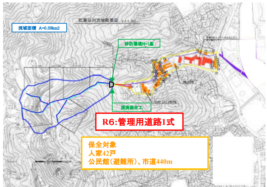
全体平面図
