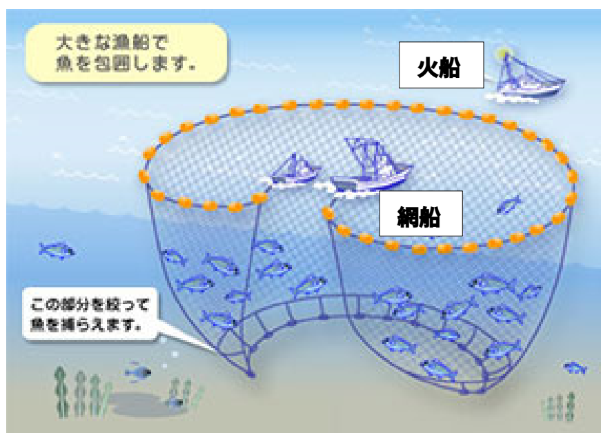
中型まき網漁業漁法図
