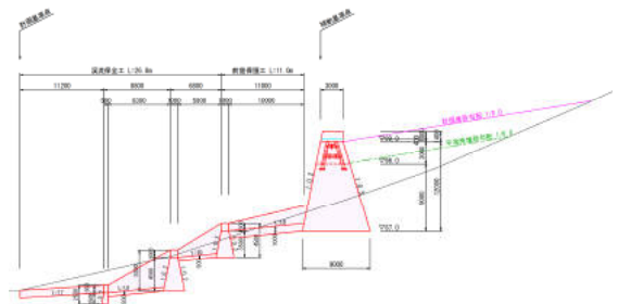
砂防堰堤側面図
