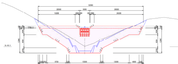
砂防堰堤正面図
