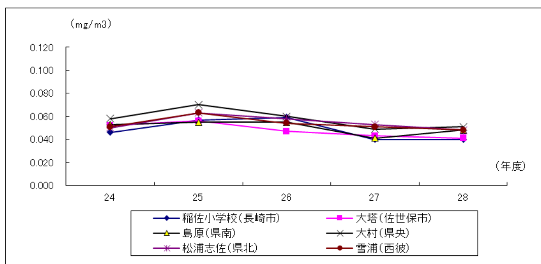
図3 浮遊粒子状物質の「年間2%除外値」の経年変化
