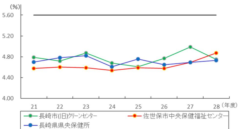
図14 1降雨時の酸性雨pH(年平均値)の経年変化
