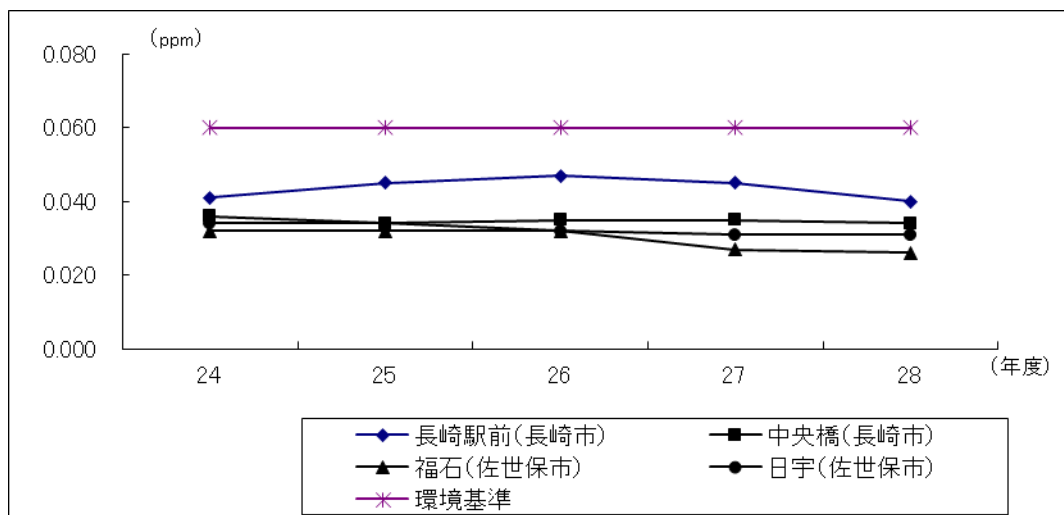
図6 二酸化窒素の「98%値」の経年変化（自動車排出ガス測定局）
