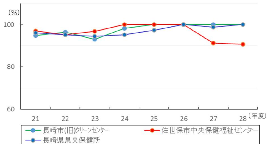
図13 1降雨時の酸性雨出現率の経年変化
