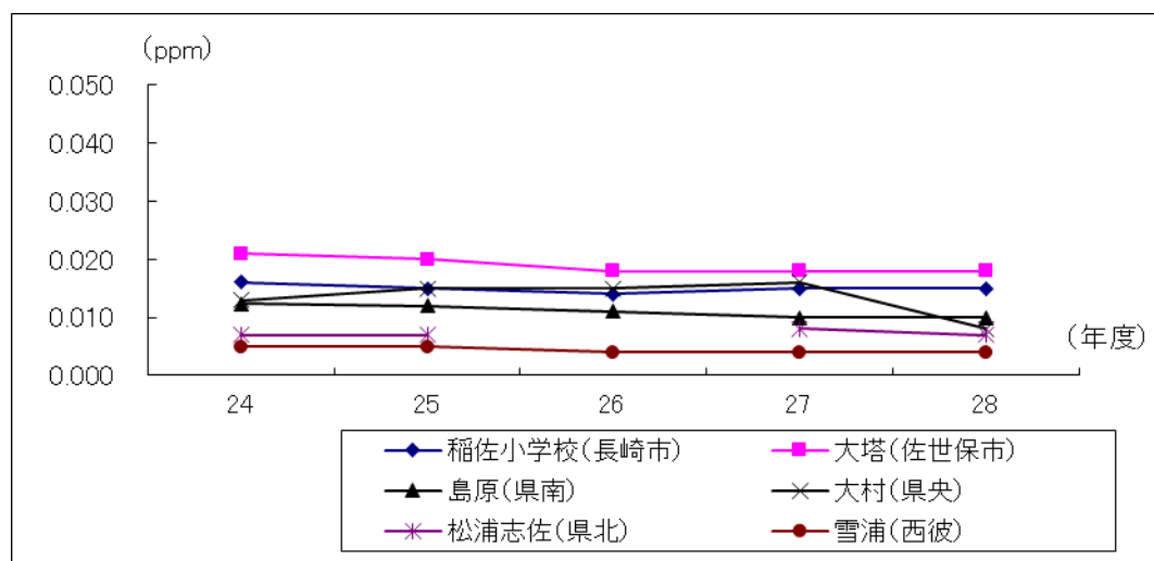
図 5 二酸化窒素の「98%値」の経年変化（一般環境大気測定局）
