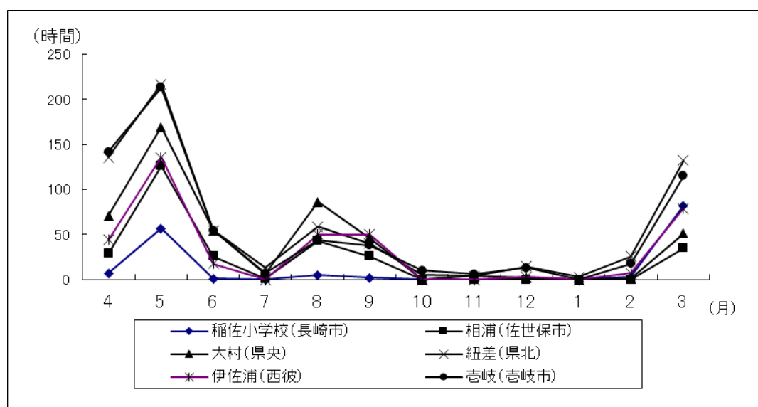
図 1 1 光化学オキシダントの環境基準月別超過状況
