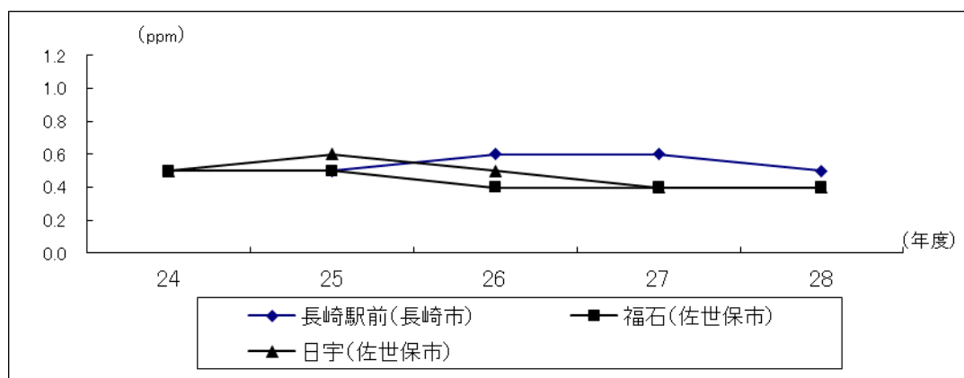
図10 一酸化炭素の「年平均値」の経年変化（自動車排出ガス測定局）
