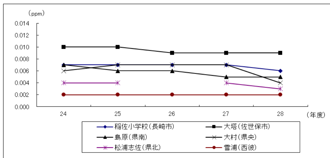
図7 二酸化窒素の年平均値の経年変化（一般環境大気測定局）
