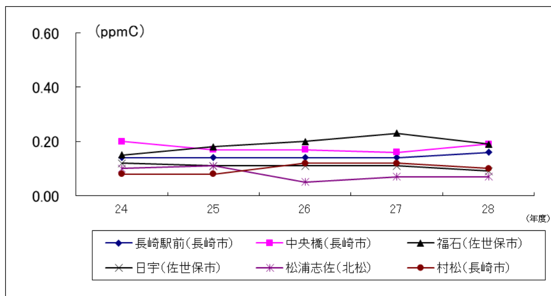
図 12 非メタン炭化水素の年平均値の経年変化
