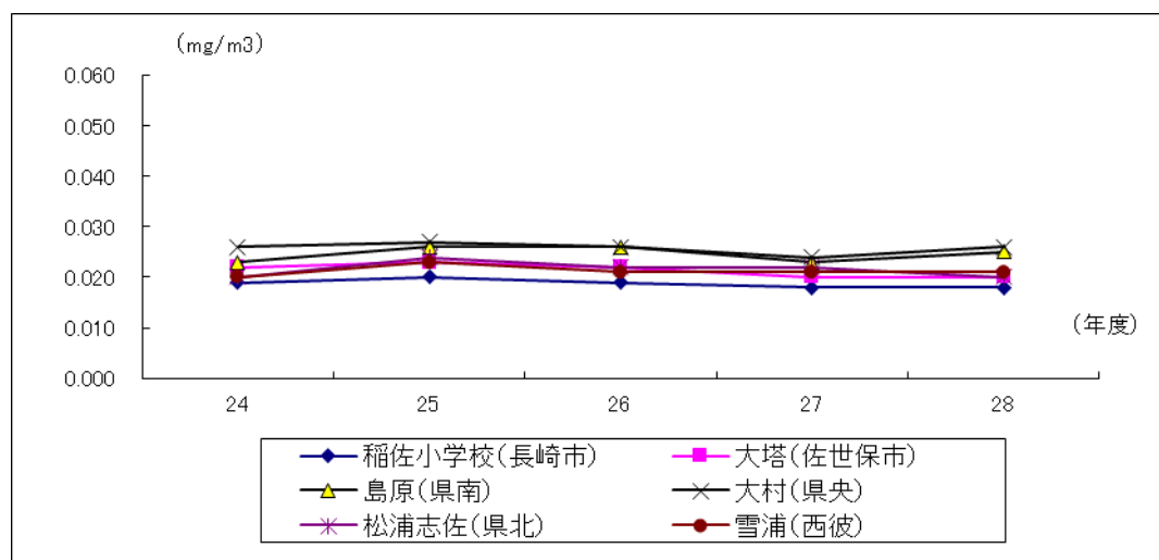
図4 浮遊粒子状物質の「年平均値」の経年変化
