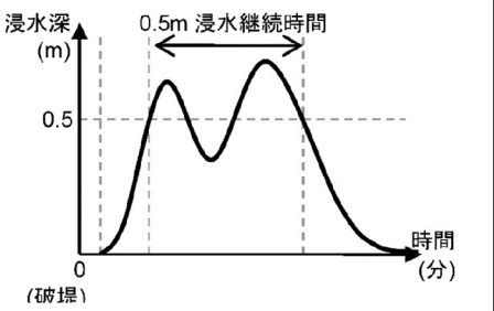
図-2 浸水継続時間
