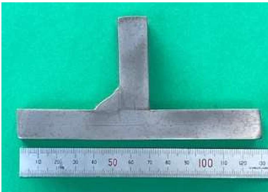
すみ肉溶接接手
