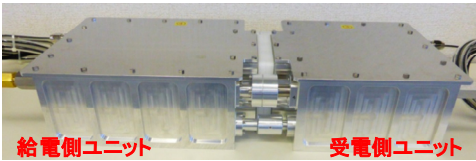
図2 非接触伝送システム（試作機）の外観
