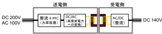
図1 電力伝送部の構成概要
