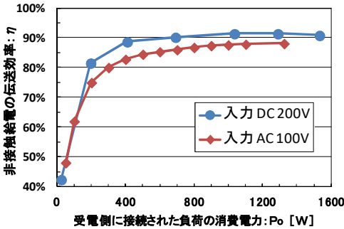
図3 負荷消費電力と伝送効率との関係
