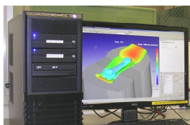
塑性加工シミュレーション
