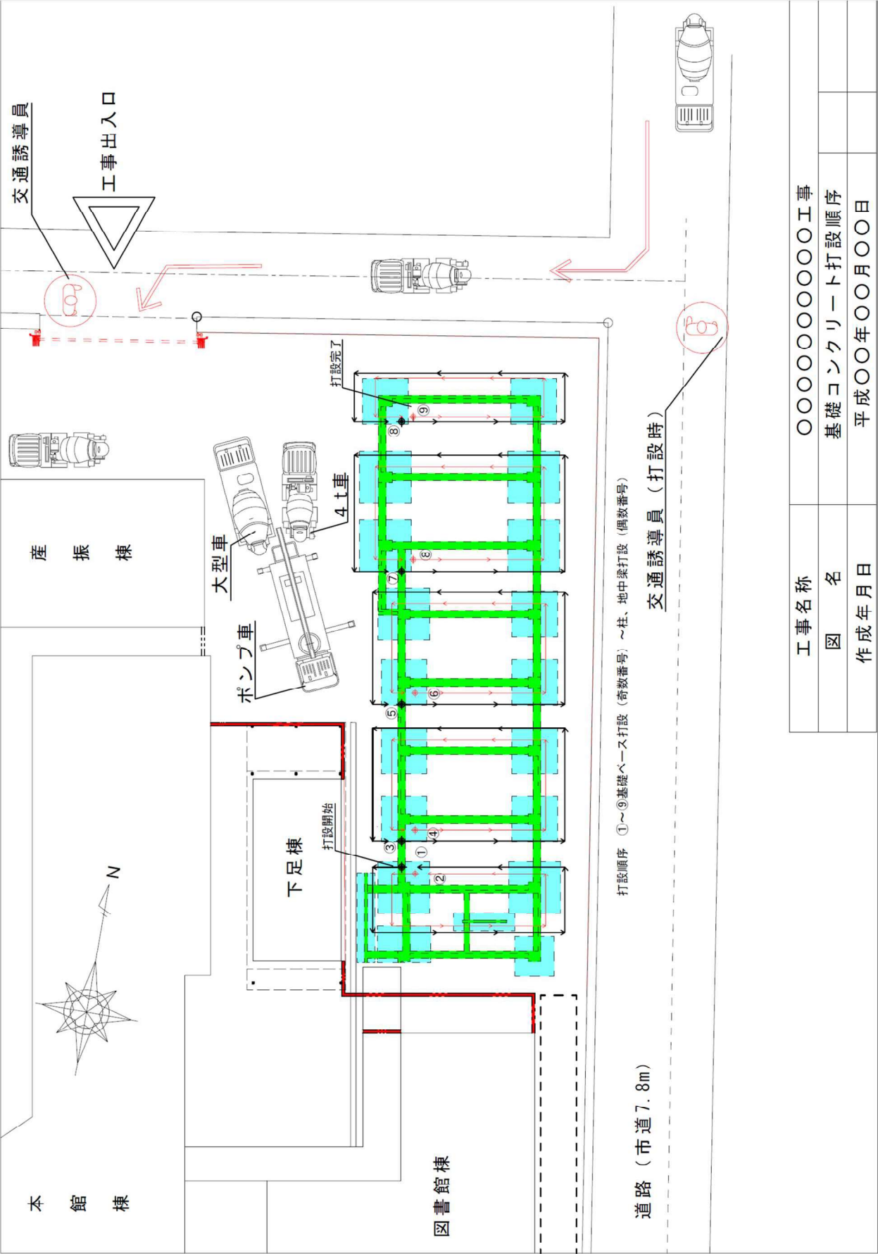
コンクリート打設計画図作成例
