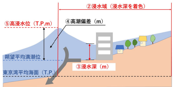
図-1 高潮浸水想定区域図における用語の定義
