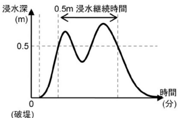
図-2 浸水継続時間
