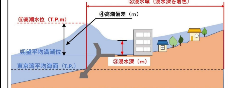
図-1 高潮浸水想定区域図における用語の定義 ②浸水域（浸水深を着色）
